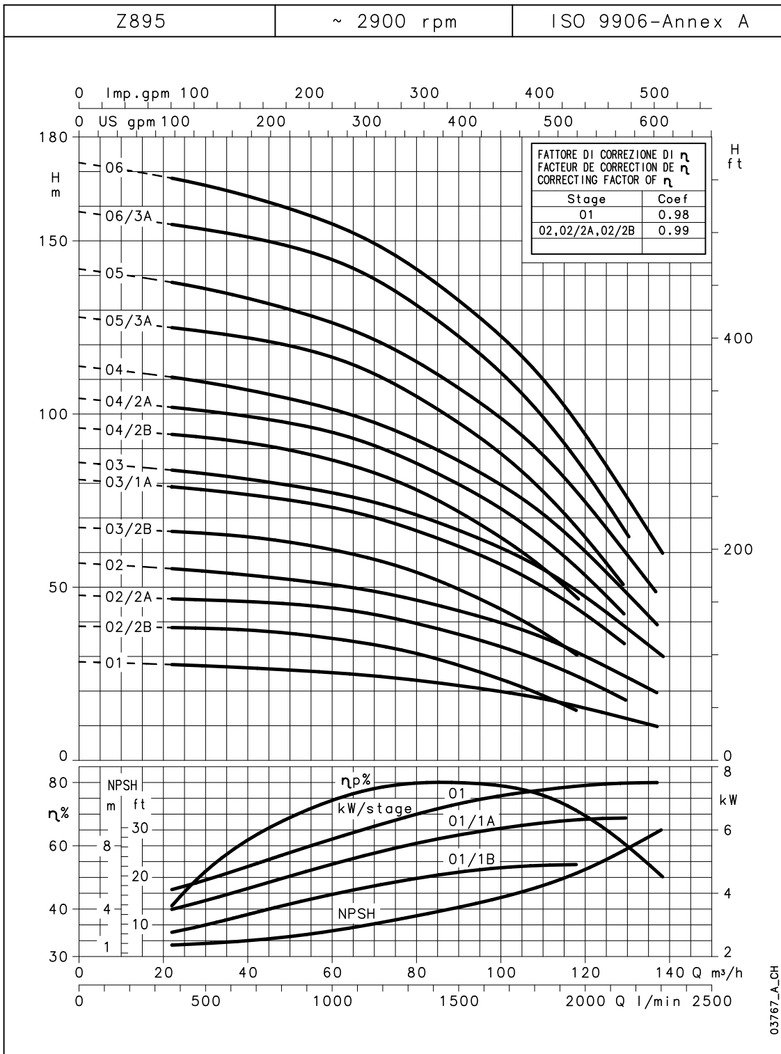
Capaciteitengrafiek Z895 serie 1-6 waaiers bij 50 Hz, 2-polig
