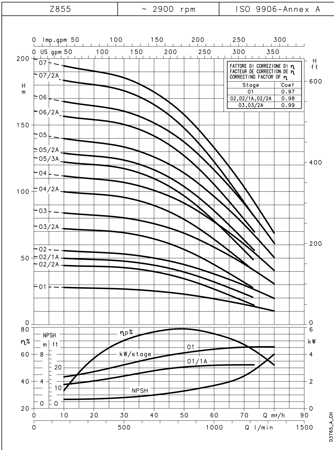
Capaciteitengrafiek Z855 serie 1-7 waaiers bij 50 Hz, 2-polig
