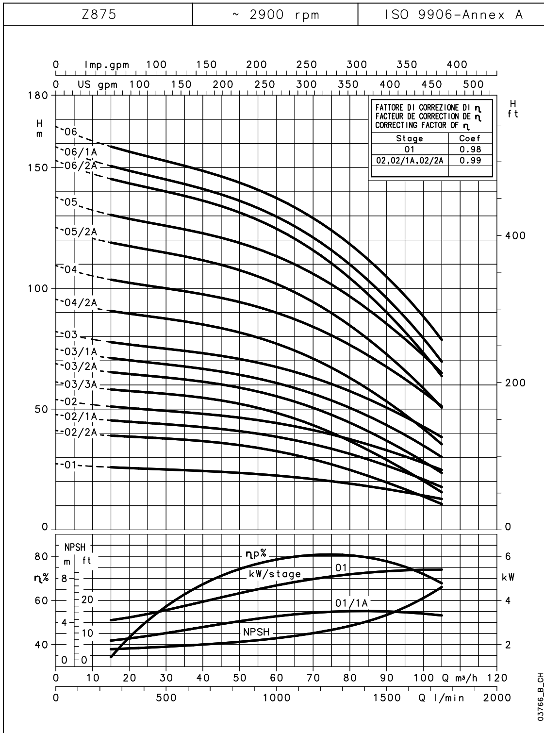
Capaciteitengrafiek Z875 serie 1-6 waaiers bij 50 Hz, 2-polig
