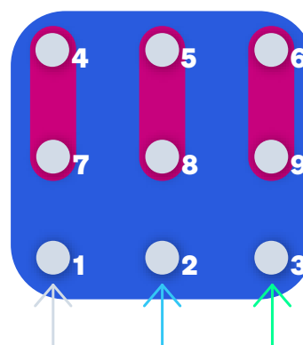
400-480 Volt 60 Hz
