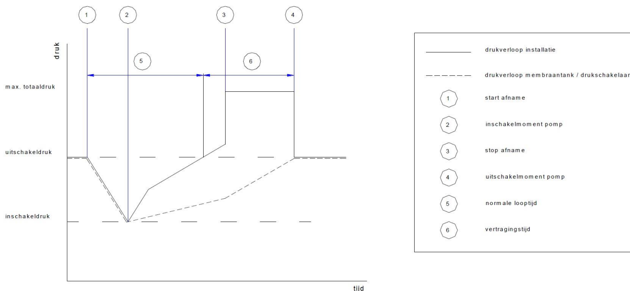
Figuur 1 Schema van vertragingstijd en de drukverloop in de installatie versus membraantank
