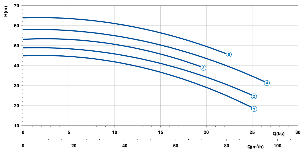
Capaciteitengrafiek D serie 50 Hz R.P.M. 2850
